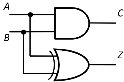
図1 半加算器
